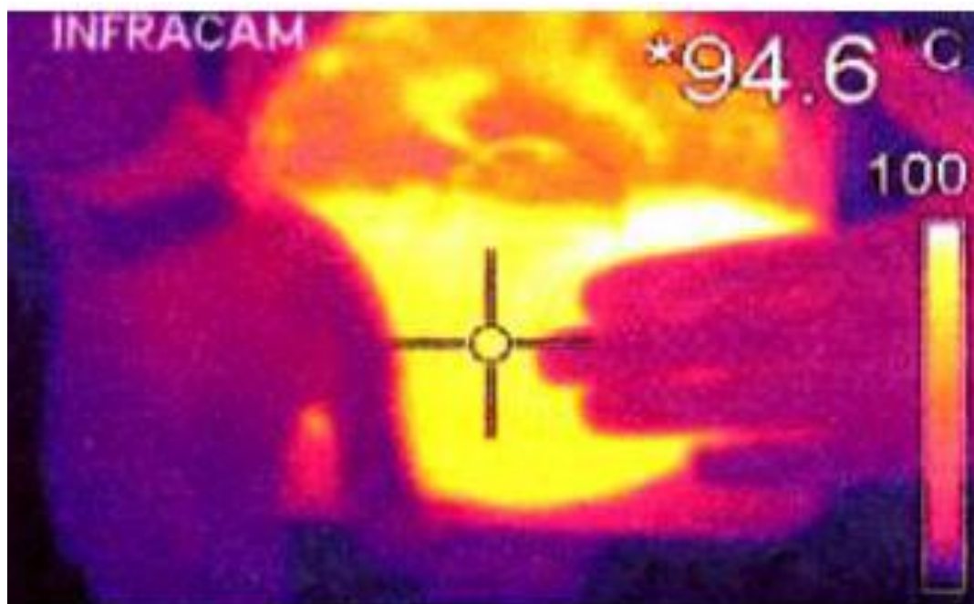
Παρουσίαση θερμογραφίας ηλεκτρικής εστίας στους 94.6 °C σε επαφή με γυμνό χέρι
